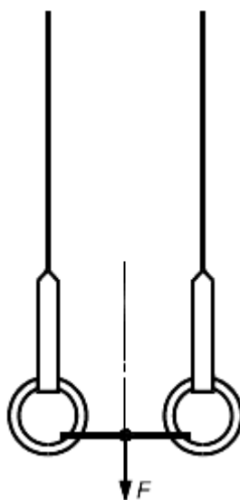
Рисунок 14 - Определение прочности закрепления гимнастических колец 10.14.2.2 Определение результатов
