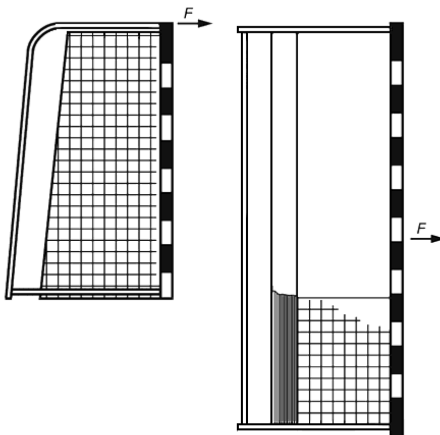
Рисунок 12 - Проверка стабильности ворот для мини-футбола
