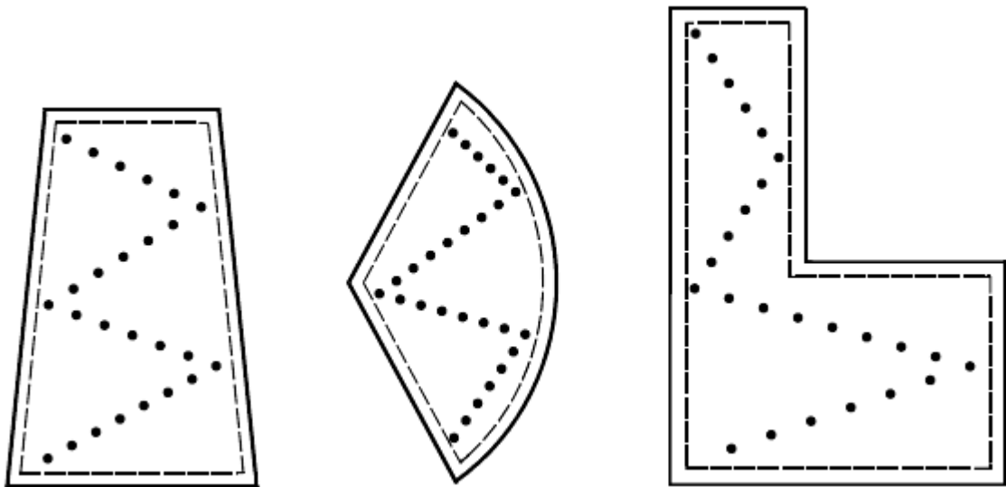
Рисунок 1 - W-образное распределение мест проведения измерений
