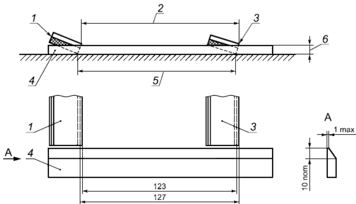
Рисунок 7 - Устройство регулировки длины пятна контакта
