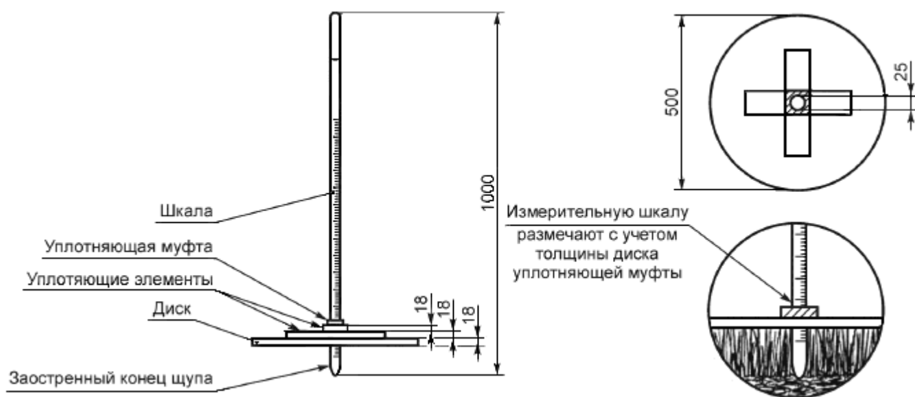
Рисунок 2 - Измерительный диск
