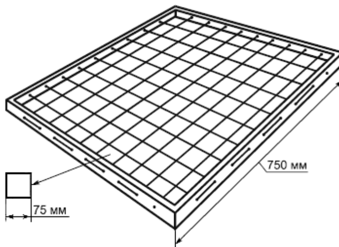
Рисунок 3 - Рама для измерения плотности травяного покрова
