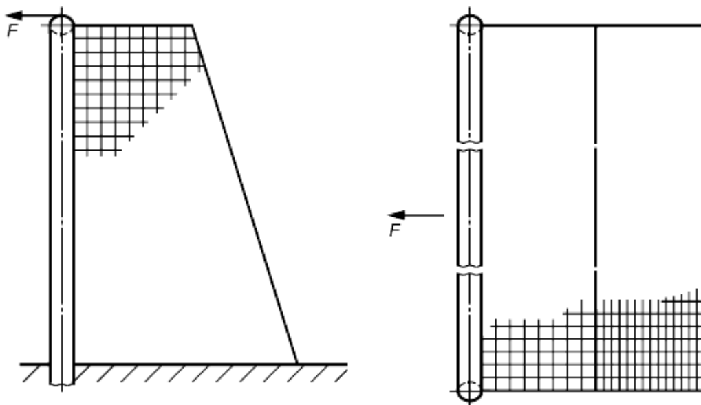
Рисунок 11 - Проверка стабильности ворот для футбола
