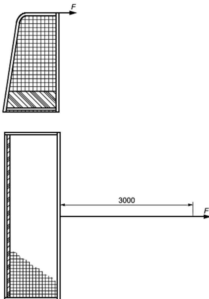
Рисунок Б.1 - Схема нагружения ворот
