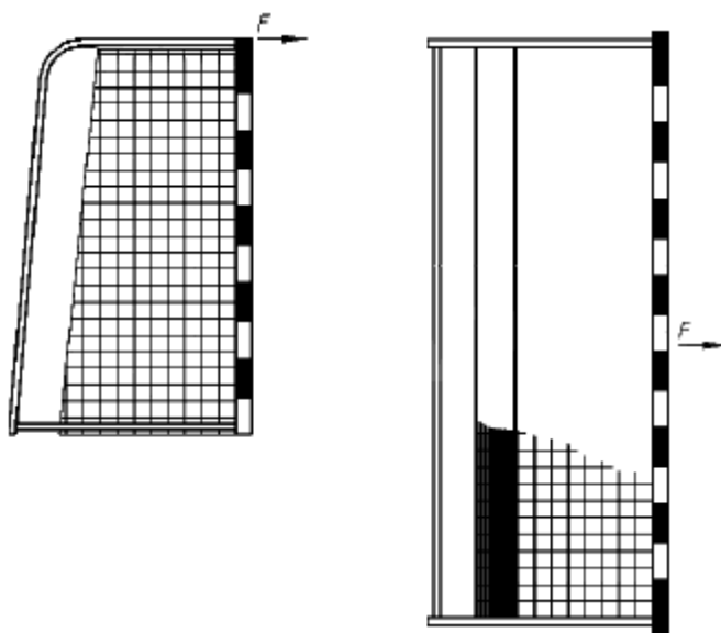
Рисунок Б.1 - Схема нагружения ворот
