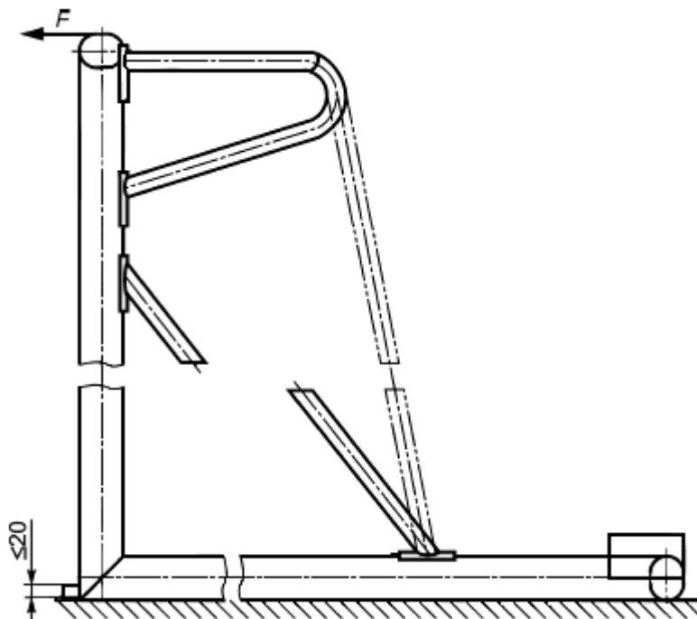
Рисунок Б.2 - Схема нагружения ворот
