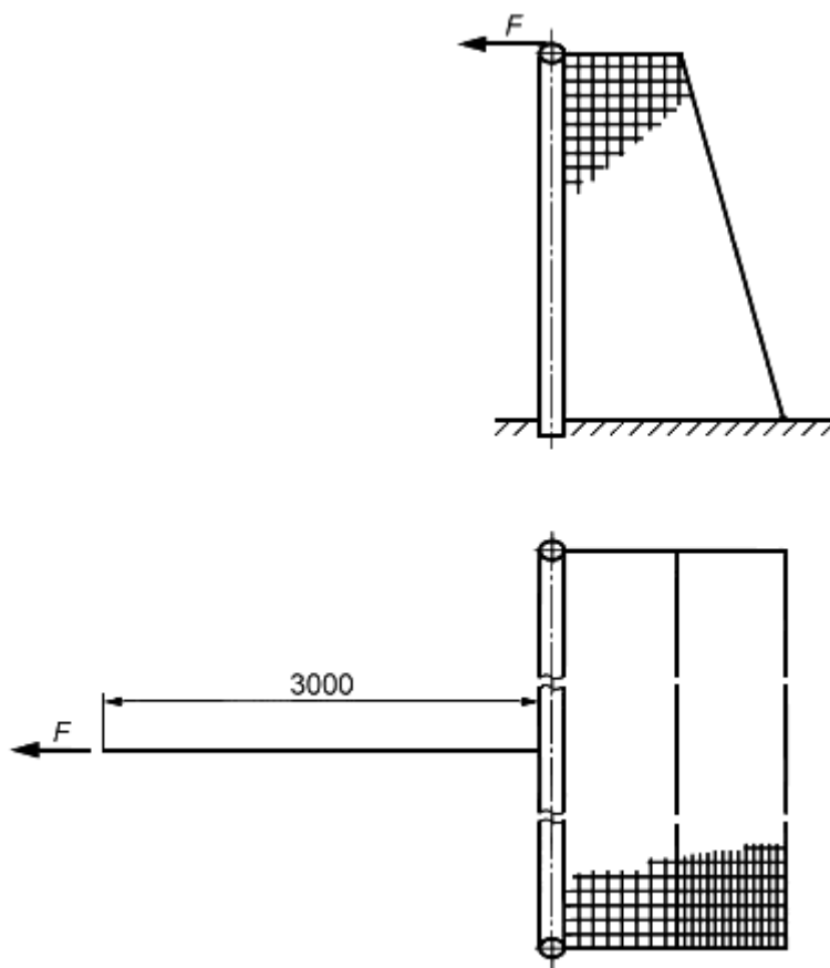
Рисунок Б.1 - Схема нагружения ворот
